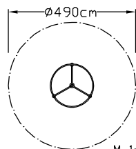
Hängekarussell KS 4033.00 >
