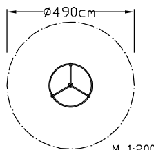
Hängekarussell KS 4033.00 >
